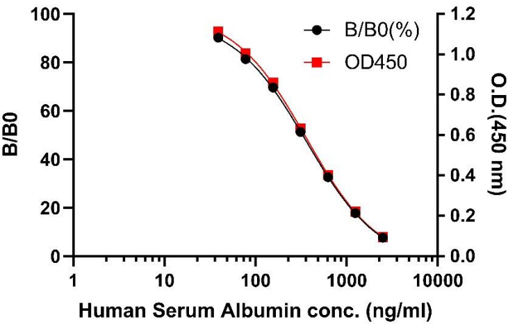
标准曲线式例
